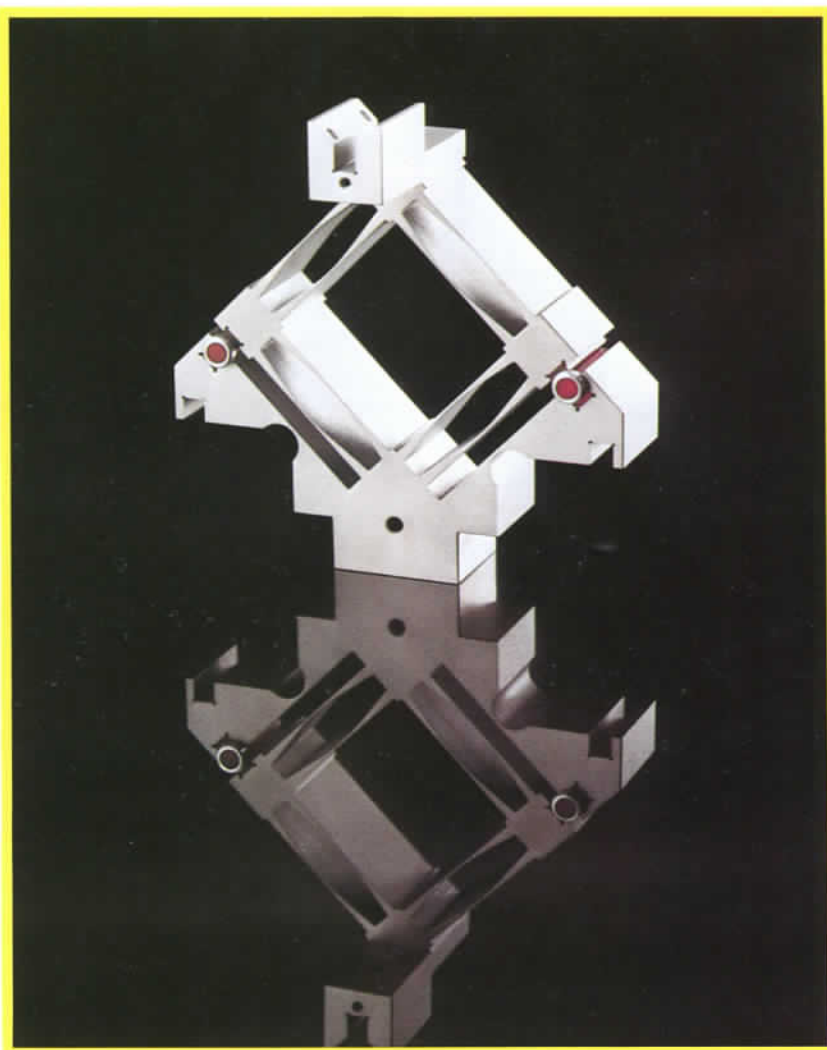
Solide déformable dans un plan permettant d'aligner 2 fibres optiques. Précision relative : 0,02 microns. photo Studio Perret.
